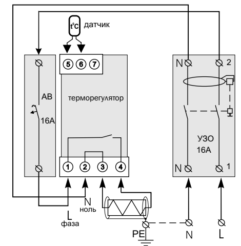
Схема 2. Подключение автоматического выключателя и УЗО
